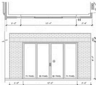
D SLIDING DOOR (OPT.)
