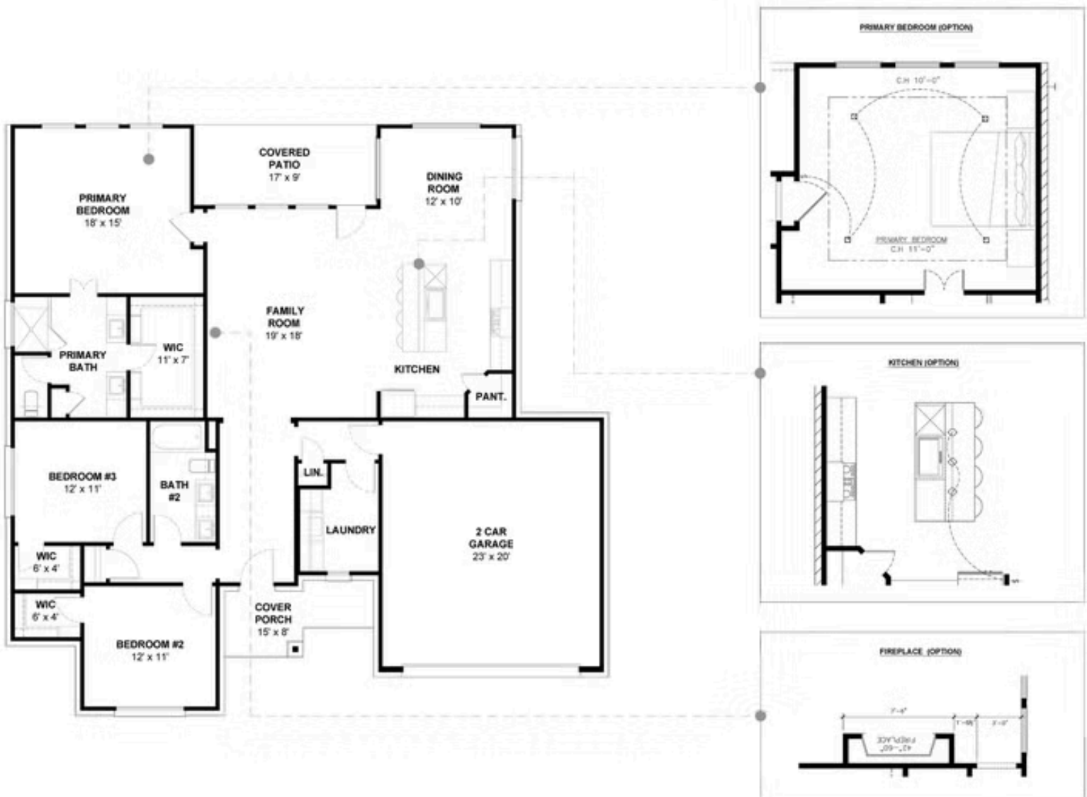
1853 Elevation B
